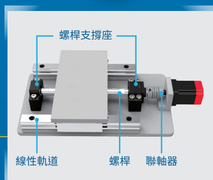
螺桿支撐座 GBK (固定端)
